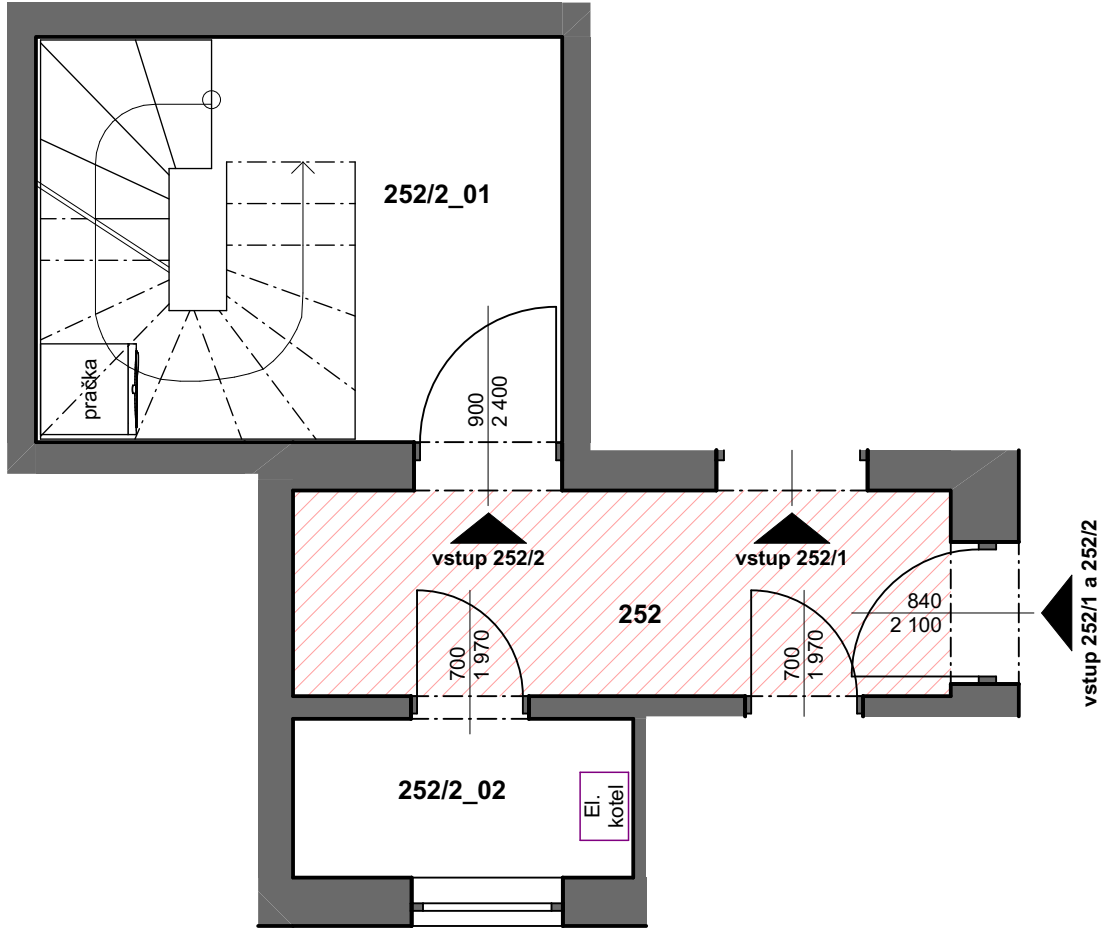
VÝSEK PŮDORYSU 1.NP
