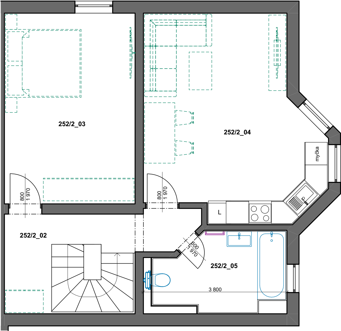
VÝSEK PŮDORYSU 2.NP
